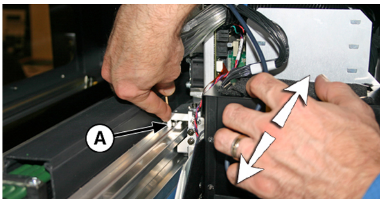
图 10-14 托架轮的位置
