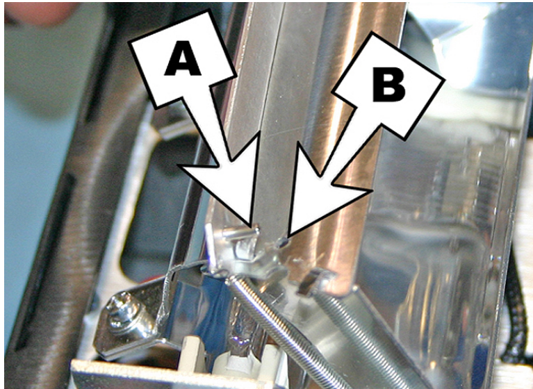
图 10-36 将销钉装入反光镜中
