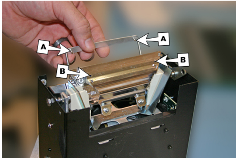
图 10-32 装有弹簧的灯
