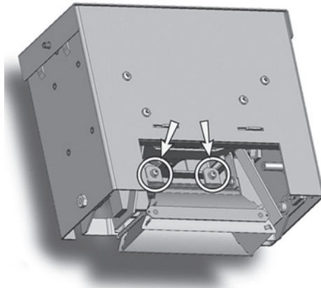
图 10-33 反光镜螺钉
