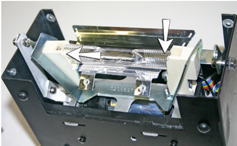
图 10-35 安装灯泡
