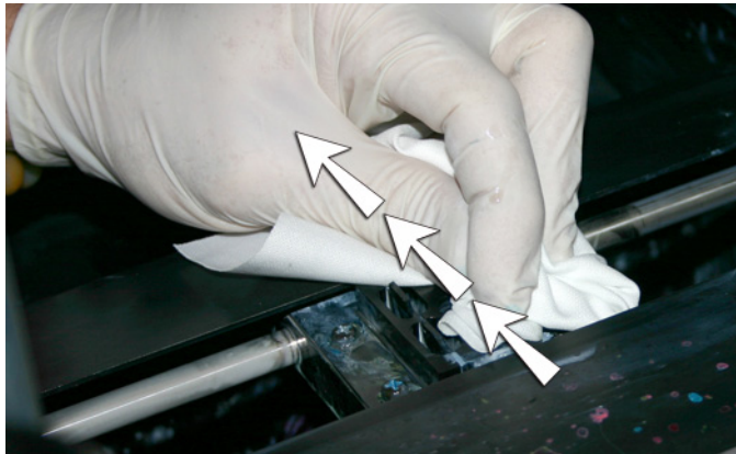
图 10-12 服务站擦拭器刀片
