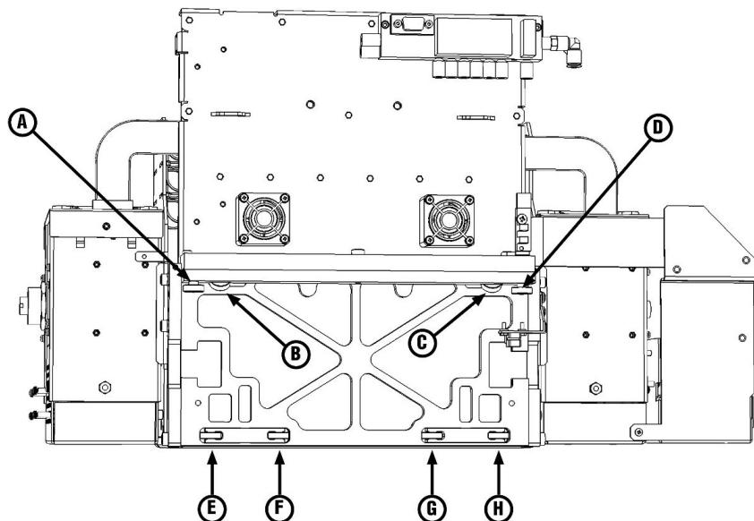
图 10-13 托架轮的位置
