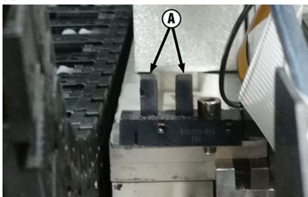
图 10-8 托架原位传感器的详细视图
