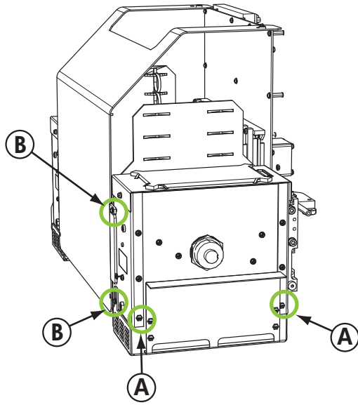
图 10-29 用户端螺钉
