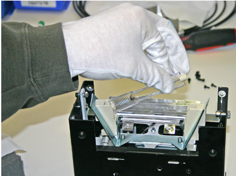
图 10-34 取下灯泡
