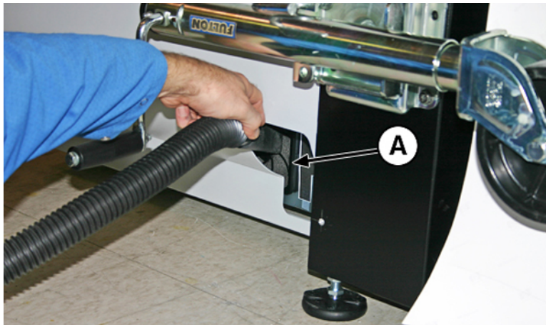
图 10-18 清洁输入端的电子设备盒风扇过滤器
