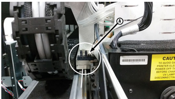
图 10-7 托架原位传感器位置
