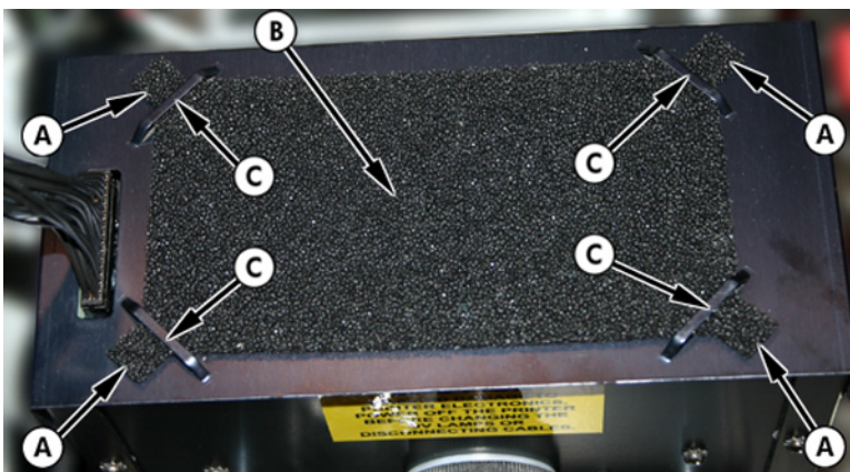
图 10-17 灯空气过滤器
