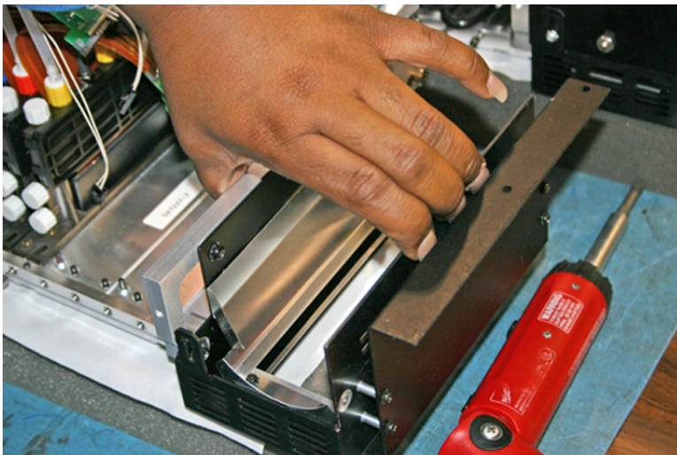
图 10-38 挤压下部灯组合件的一侧
