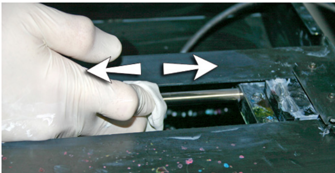
图 10-11 清洁导轨
