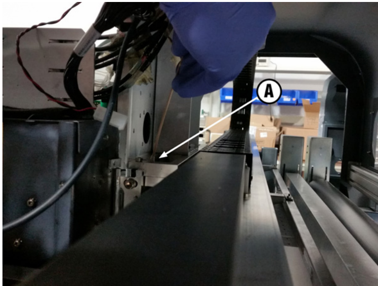
图 10-16 用棉签清洁倾斜托架轮 (2 / 2)
