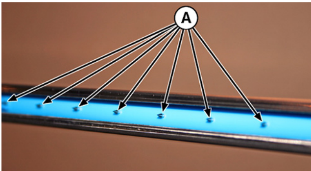
图 10-23 离子发生器针
