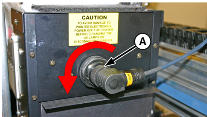
图 10-28 灯的电源线
