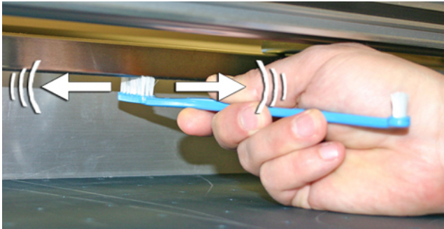
图 10-22 用附带的毛刷清洁离子发生器针
