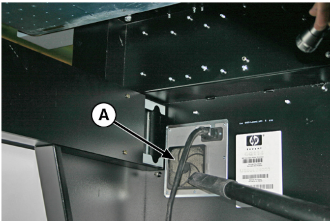
图 10-19 吸除电子设备盒风扇过滤器的灰尘
